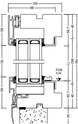
Schnitt senkrecht
