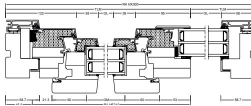
Schnitt waagrecht mit eingebautem Fenster
